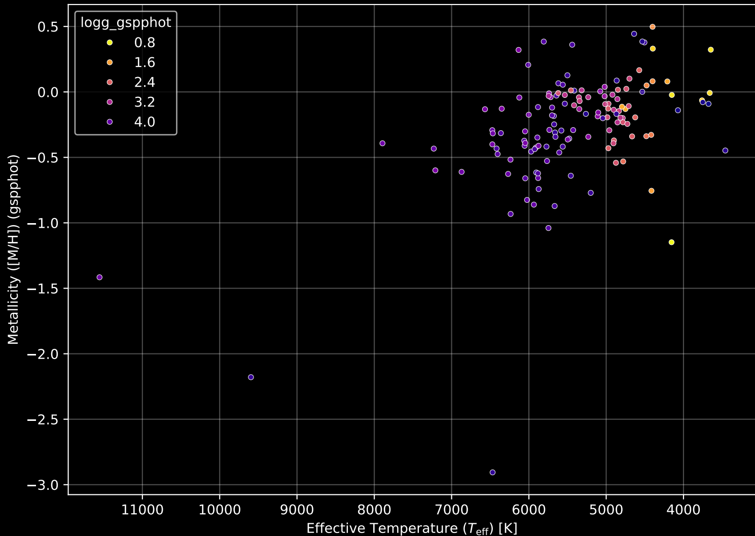
APOGEE DR17 Field: [275-34-O_TESS] Stellar Population Parameters (n= 137)
